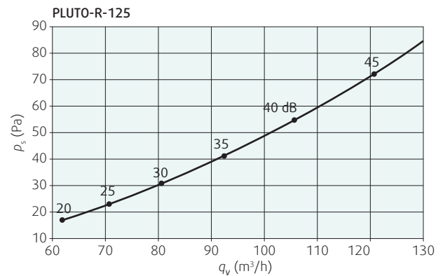
Graf 1: Tlaková strata a A-vážená hladina akustického výkonu
