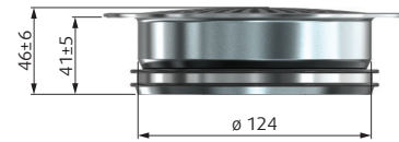
Obr. 1: Rozmery difúzora PLUTO
