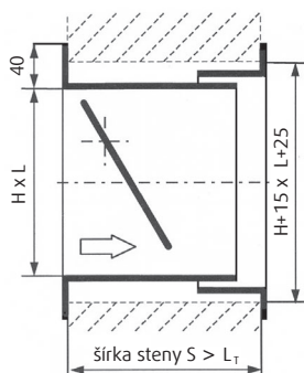
Stenové vyhotovenie „W“ Pri šírke steny S > L_T
