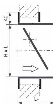
Stenové vyhotovenie „T“ Pri šírke steny S \leq L_T
