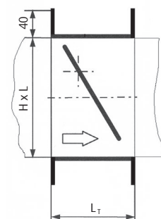
Potrubné vyhotovenie „D“
