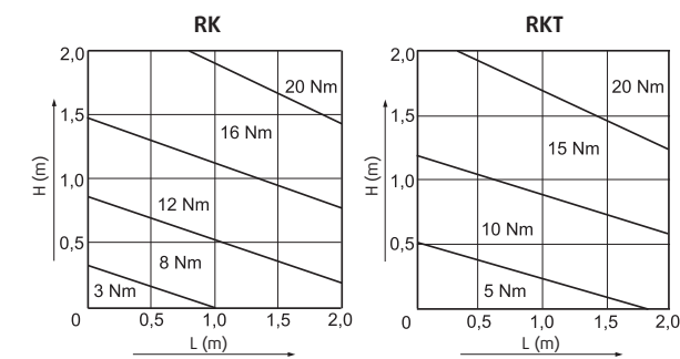
Graf 1: Veľkosť krútiaceho momentu pre servopohony
